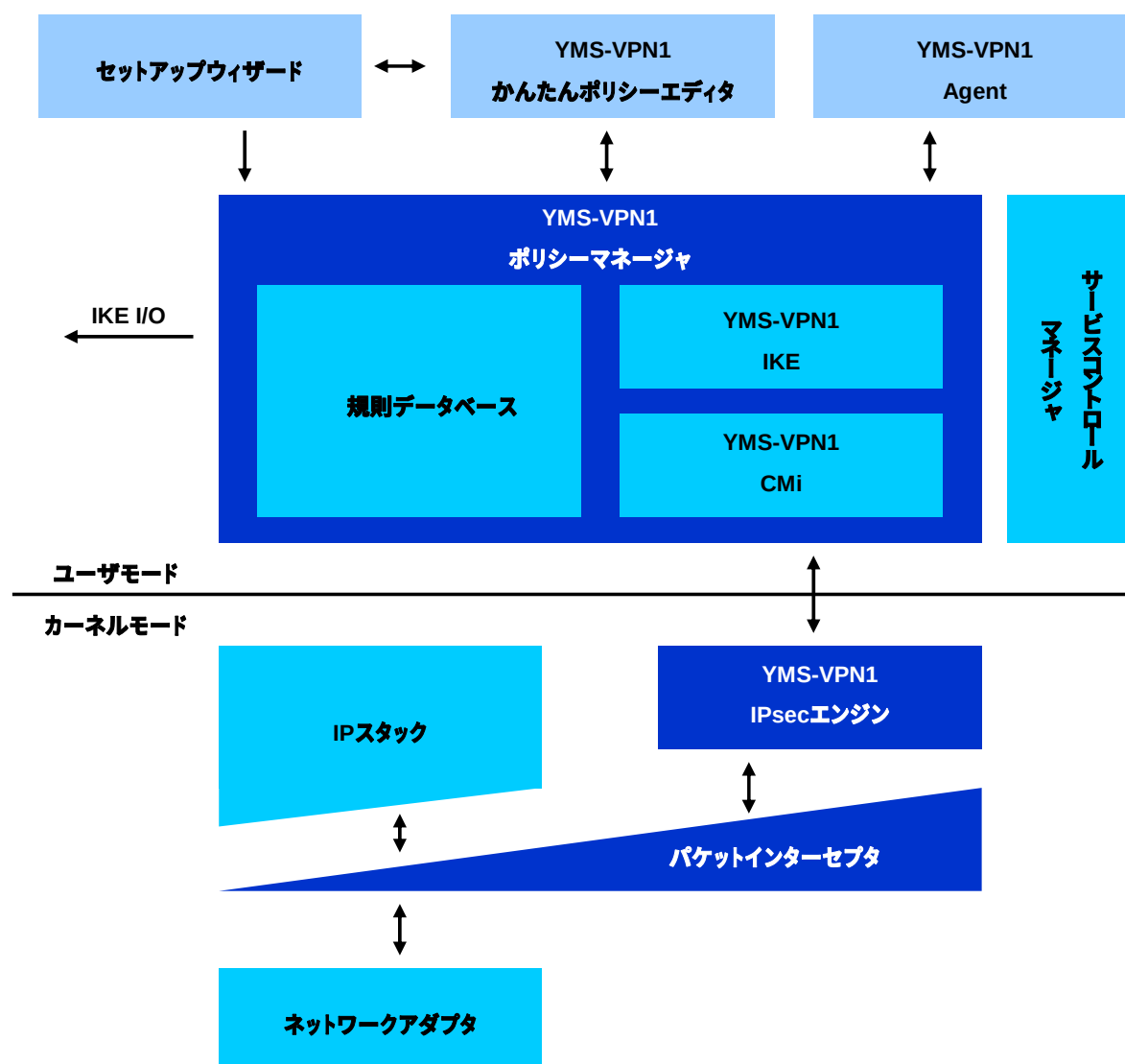
図 3-1 ソフトウェアの詳細なアーキテクチャ
